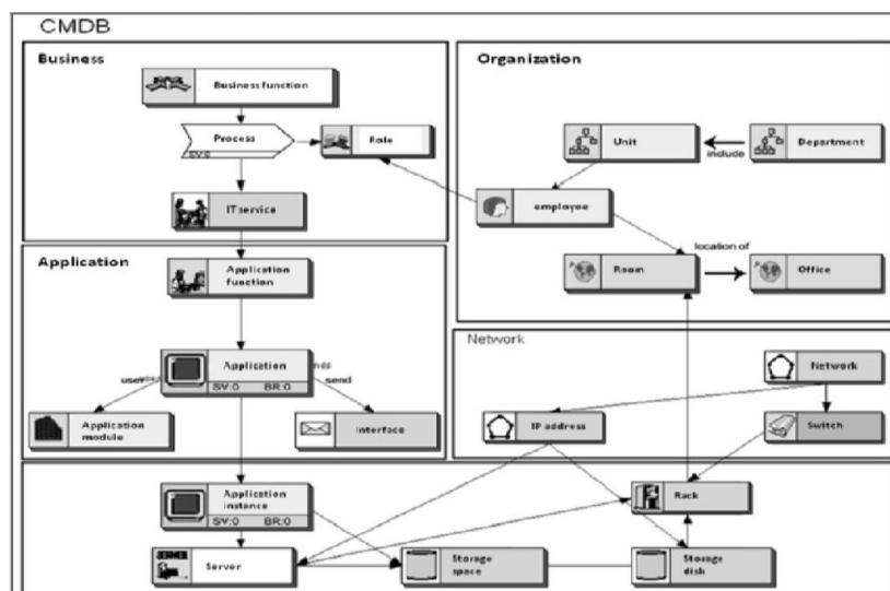
Рис. 6.24. Модель данных
