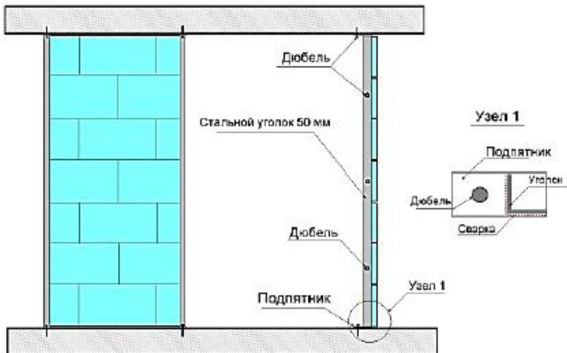
Рисунок 26. Конструкция мелкоблочной перегородки.
