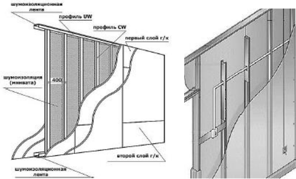
Рисунок 25. Конструкция каркасной перегородки.
