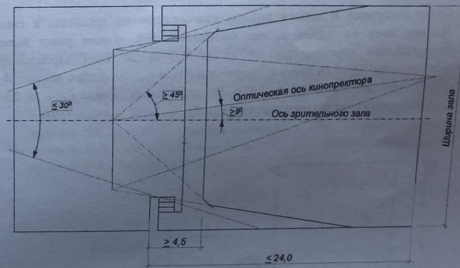
Рис. 8. Размещение зрительских мест, расположение и размеры экрана.
