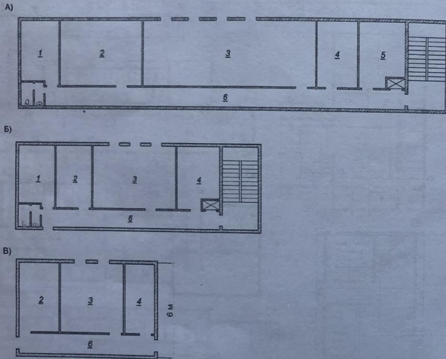
Рис. 12. Планы киноаппаратных: А- широкоформатного кинотеатра; Б- широкоэкранного кинотеатра; В- сезонного кинотеатра; 1- комната кинотехника; 2- аппаратная; 3- кинопроекционная; 4- перемоточная; 5- мастерская; 6- коридор
