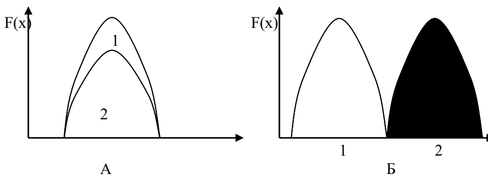
Рис. 1. Изменение функции отклика (выживаемости) вида в зависимости от изменения фактора
