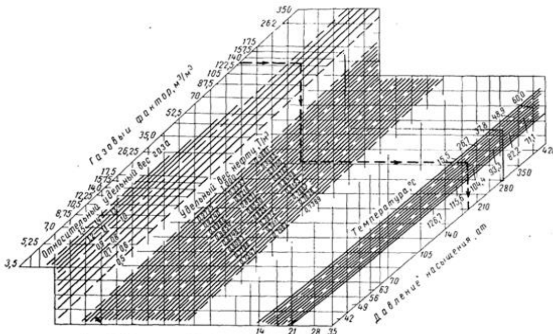
Рис. 1. Номограмма М. Стендинга для определения давления насыщения.
