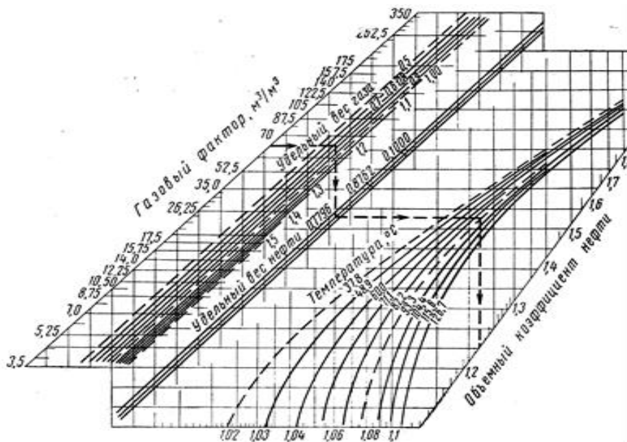
Рис. 2 Номограмма для определения объемного коэффициента нефти при давлении насыщения
