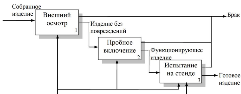
Рис. 5.7. Фрагмент диаграммы декомпозиции работы «Контроль качества»
