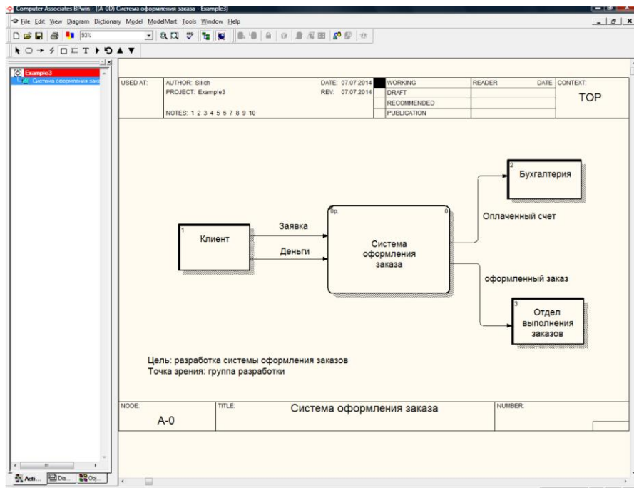
Рис. 4.1. Контекстная диаграмма в нотации DFD
