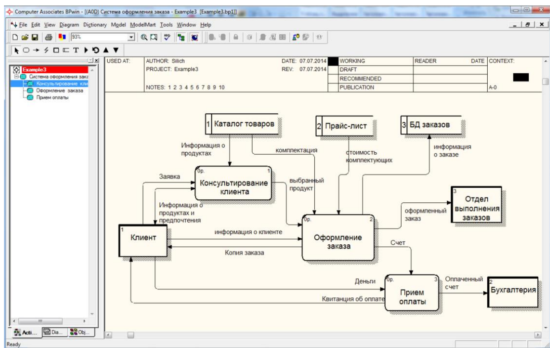
Рис 4.3. Декомпозиционная DFD-диаграмма
