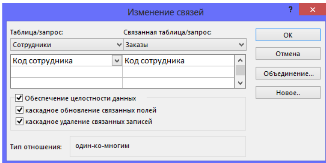
Рис. 1. Создание связи между таблицами
