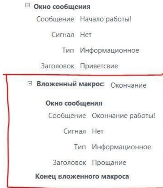
Рис. 4. Аргументы для макроса ОкноСообщения
