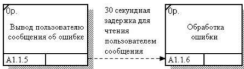
Рисунок 4 – Связь типа «отношение»
