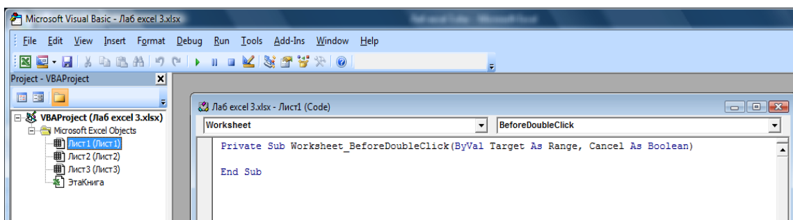
Рис. 14. Процедура Worksheet_BeforeDoubleClick
