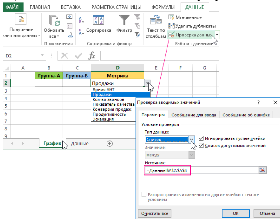
Рис.3.3 Проверка данных
