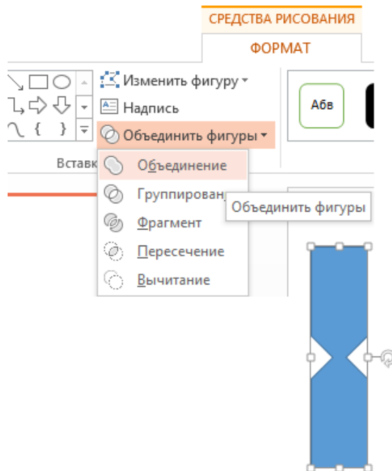
Рис.2.9 Объединение фигур
