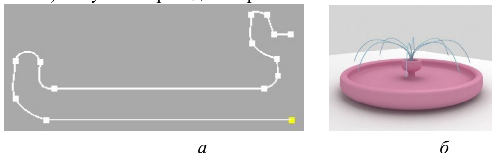
Рисунок 17. Создание фонтана
