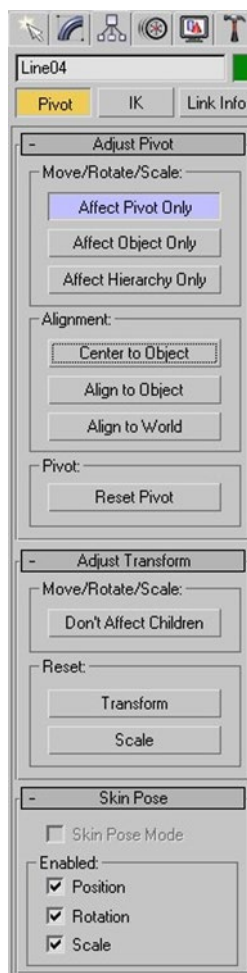
Рисунок 31. Вкладка Hierarchy
