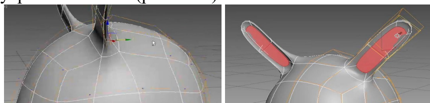
Рисунок 12. Создание ушей
