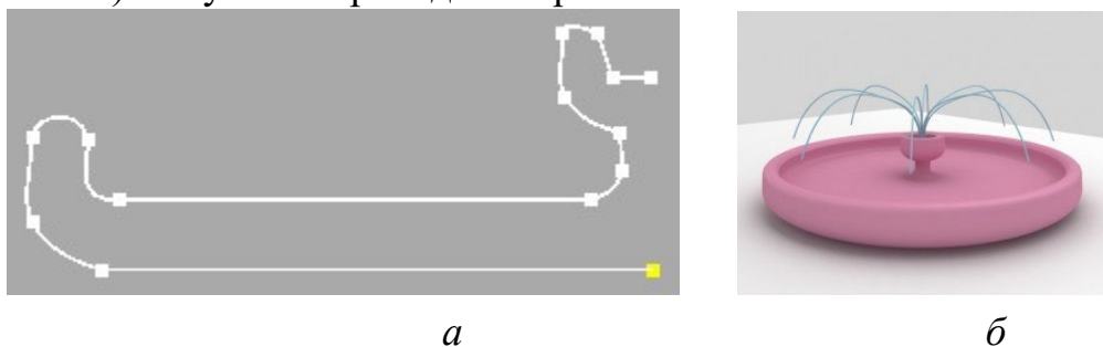
Рисунок 17. Создание фонтана
