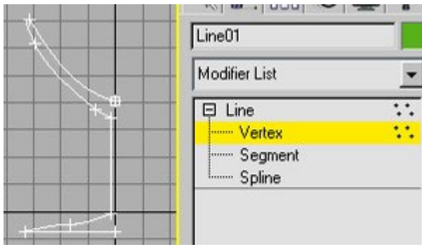
Рисунок 16. Создание фужера
