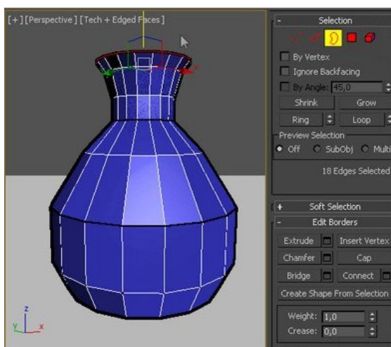
Рисунок 9. Создание вазы
