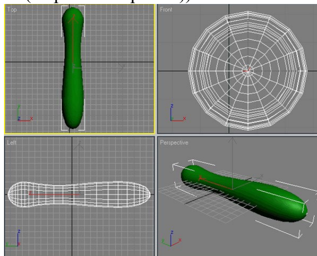
Рисунок 30. Объект после применения модификатора Lathe (Вращение вокруг оси) и задания соответствующих настроек
