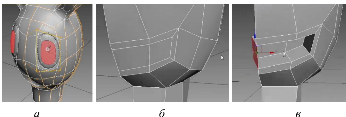
Рисунок 13. Создание деталей
