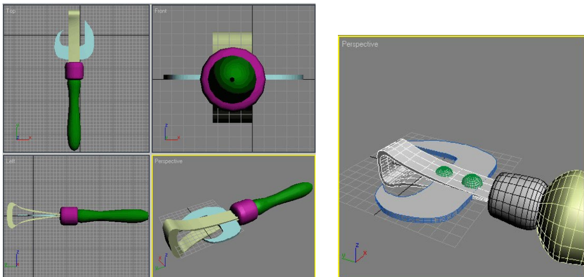
Рисунок 31. Вкладка Hierarchy
