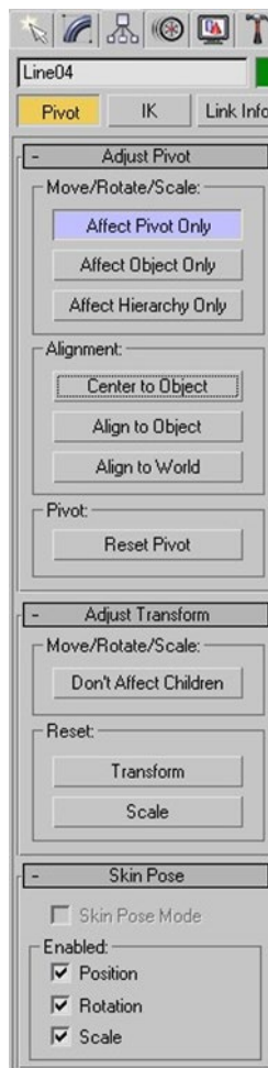
Рисунок 31. Вкладка Hierarchy
