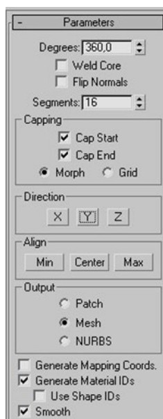
Рисунок 27. Вид окна
