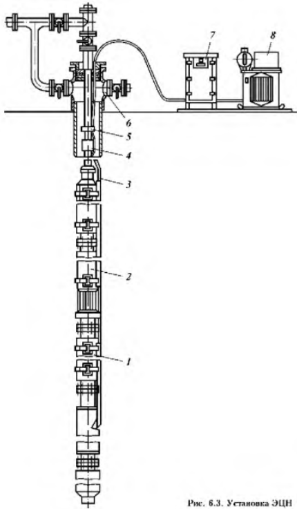
Рис. 6.3. Установка ЭЦН
