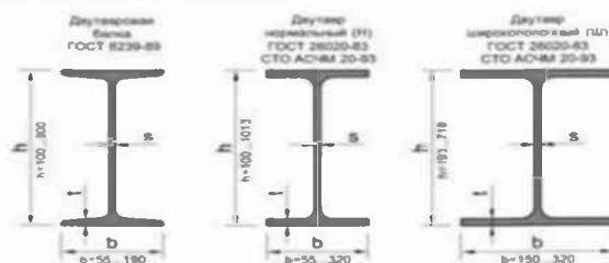
Рис. 1.2 Виды прокатных двутавров, которые используются как балки.
