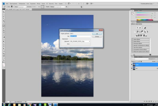
Рис 2. 2. Создание слоя
